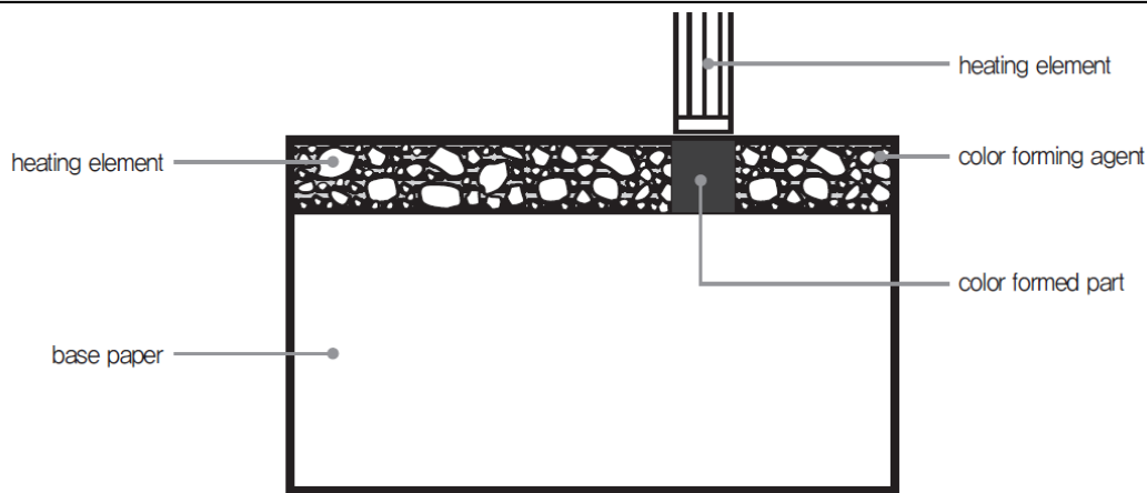
그림 16. 감열지의 구조
